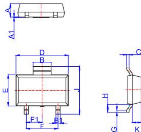
SOT-89-2L
